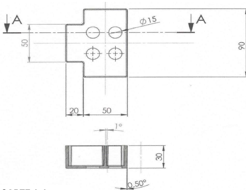
CORTE A-A
